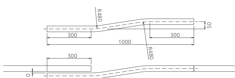
交叉レール
