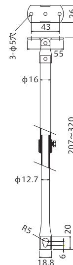
大型伸縮吊棒寸法図 (mm)
