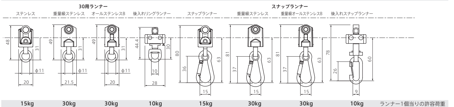
ランナー1個当りの許容荷重
