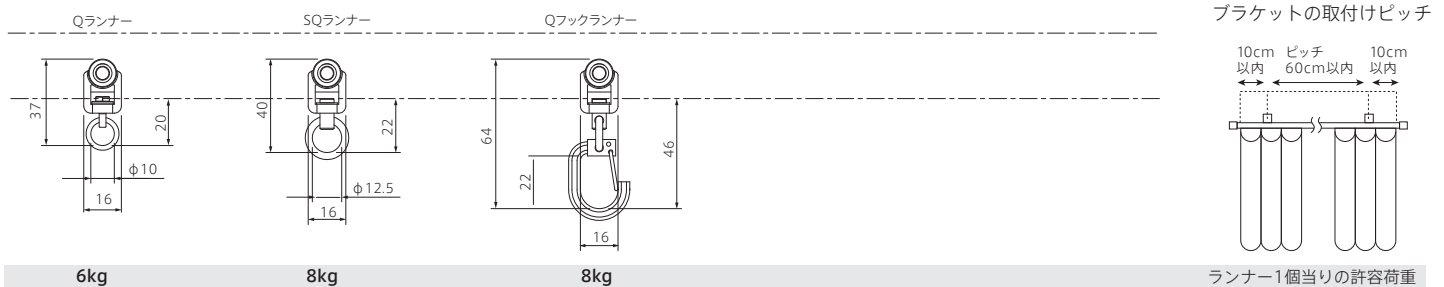
ランナー1個当りの許容荷重
