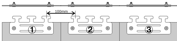
シートラップ図 (のれんシート幅200mmの場合)
